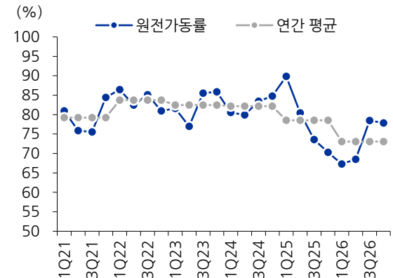
도표16. 원전가동률
